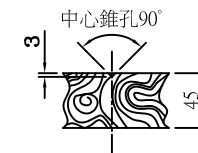
B-B剖视图
